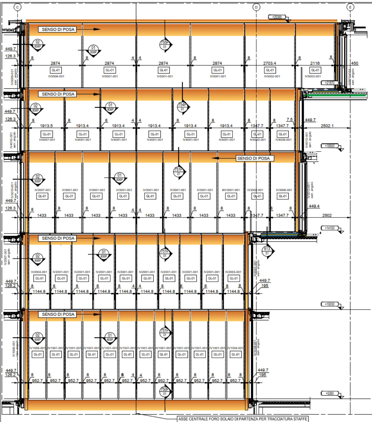
01 SEZ. VERT. Scale: 1:80
